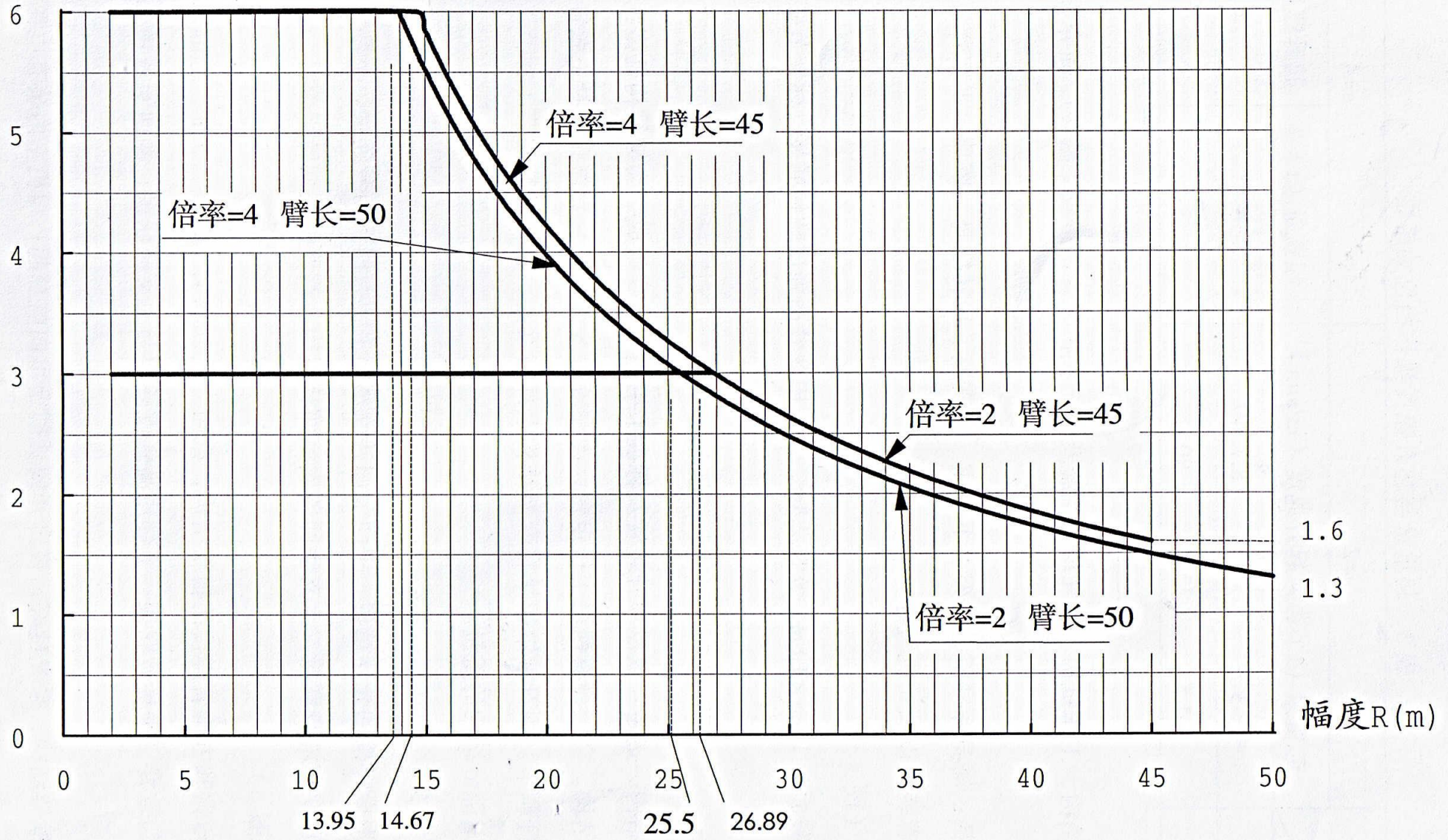
图1 起重特性曲线
